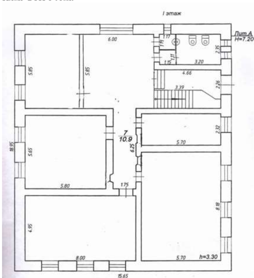
План БТИ 1 этаж
